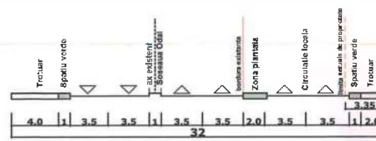
PROFIL A-A' - SOSEAU ODAI - PROFIL STRADAL PROPU, CONFORM PUZ SOS. ODAI - SOS. BUCURESTI - PLOIESTI - STRADA JANDARMERIEI - SOSEAU I. IONESCU-SISESTI - SOS. BUCURESTI - TARGOVISTE
