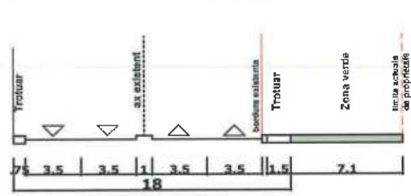
PROFIL A-A' - SOSEAU ODAI PROFIL EXISTENT
